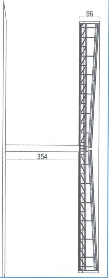
2 Corte "BB" - Intervenção 02 1/100
