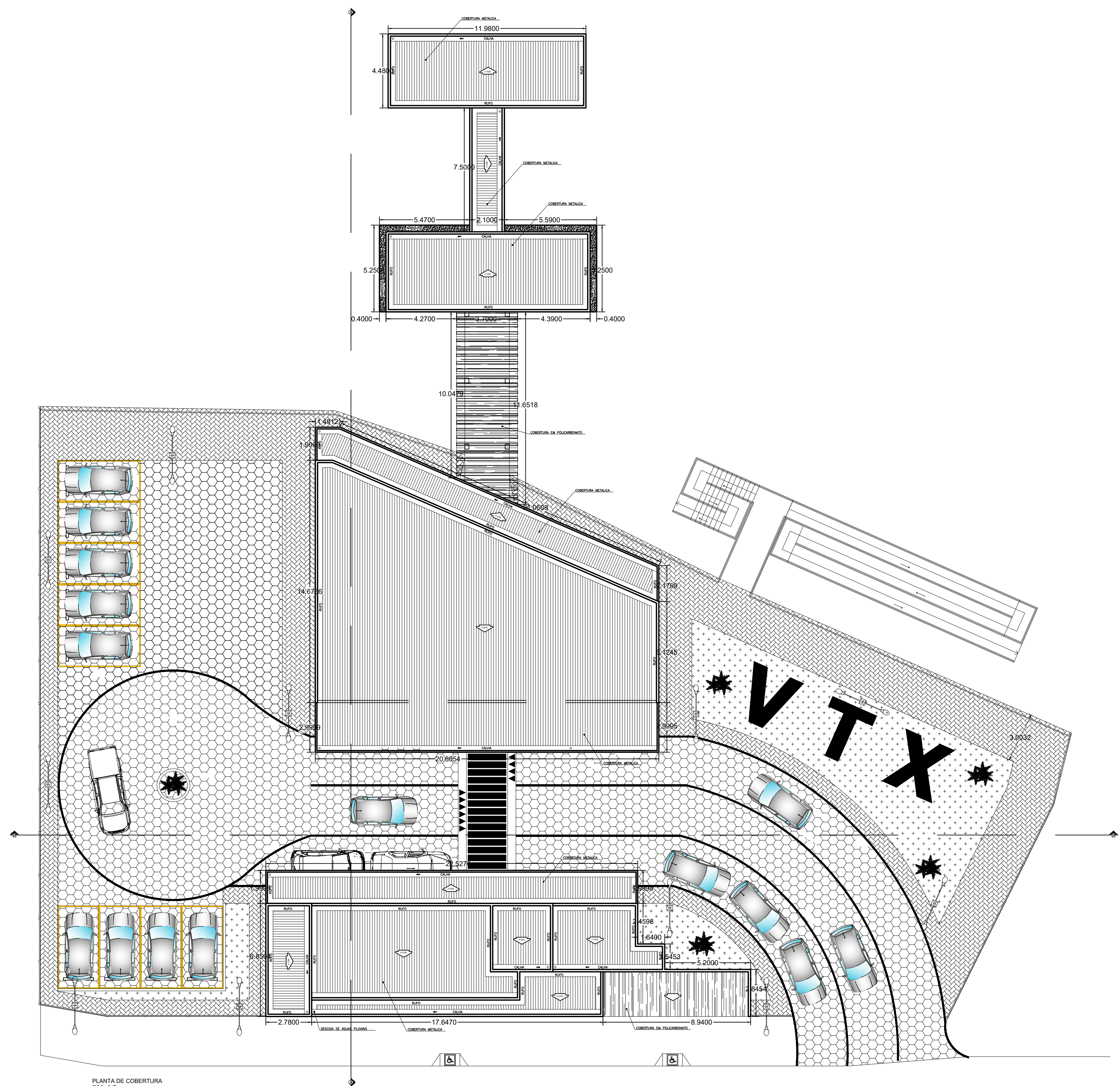
PLANTA DE COBERTURA ESC: 1/50
