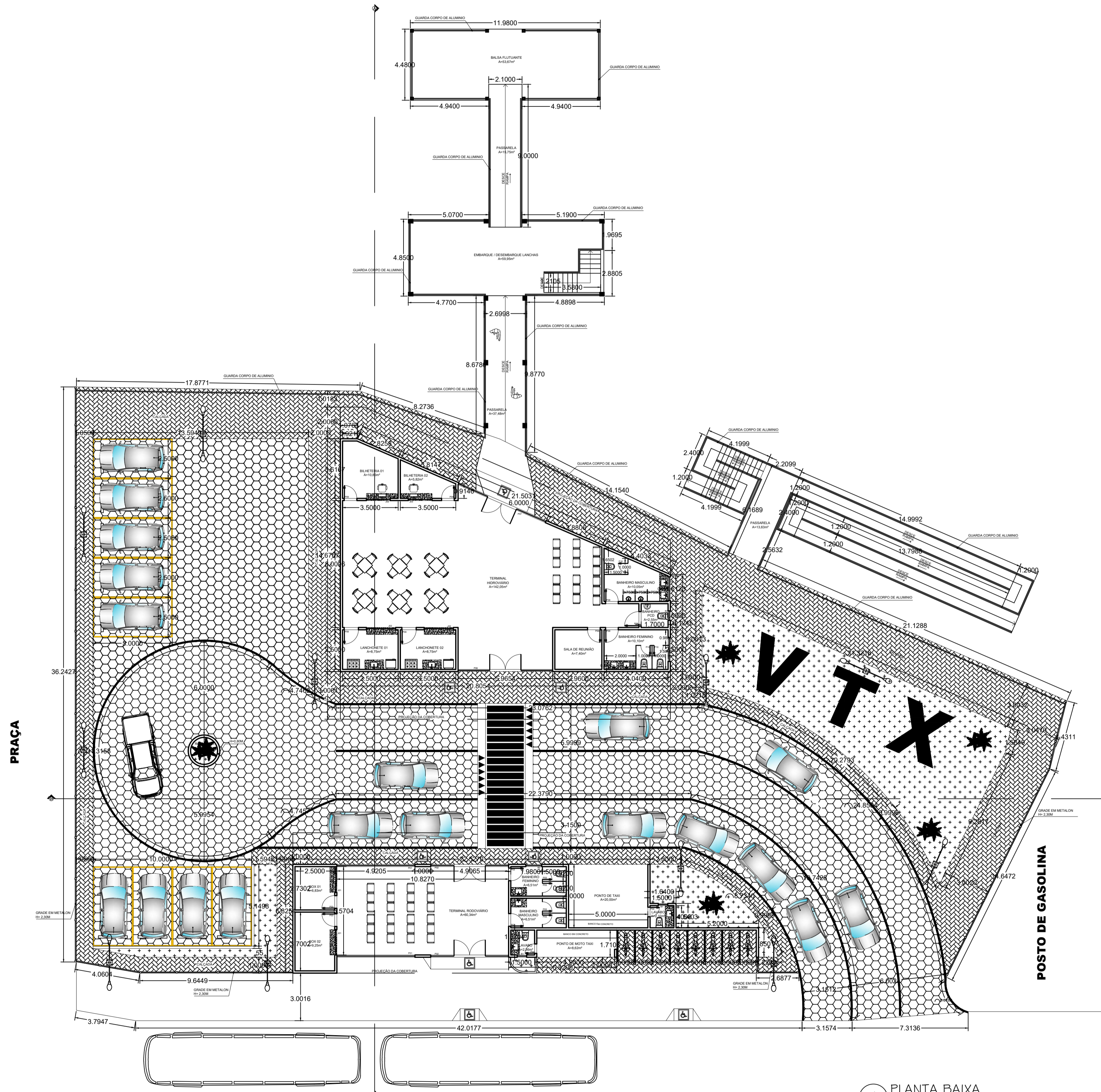
PLANTA BAIXA 1/150
