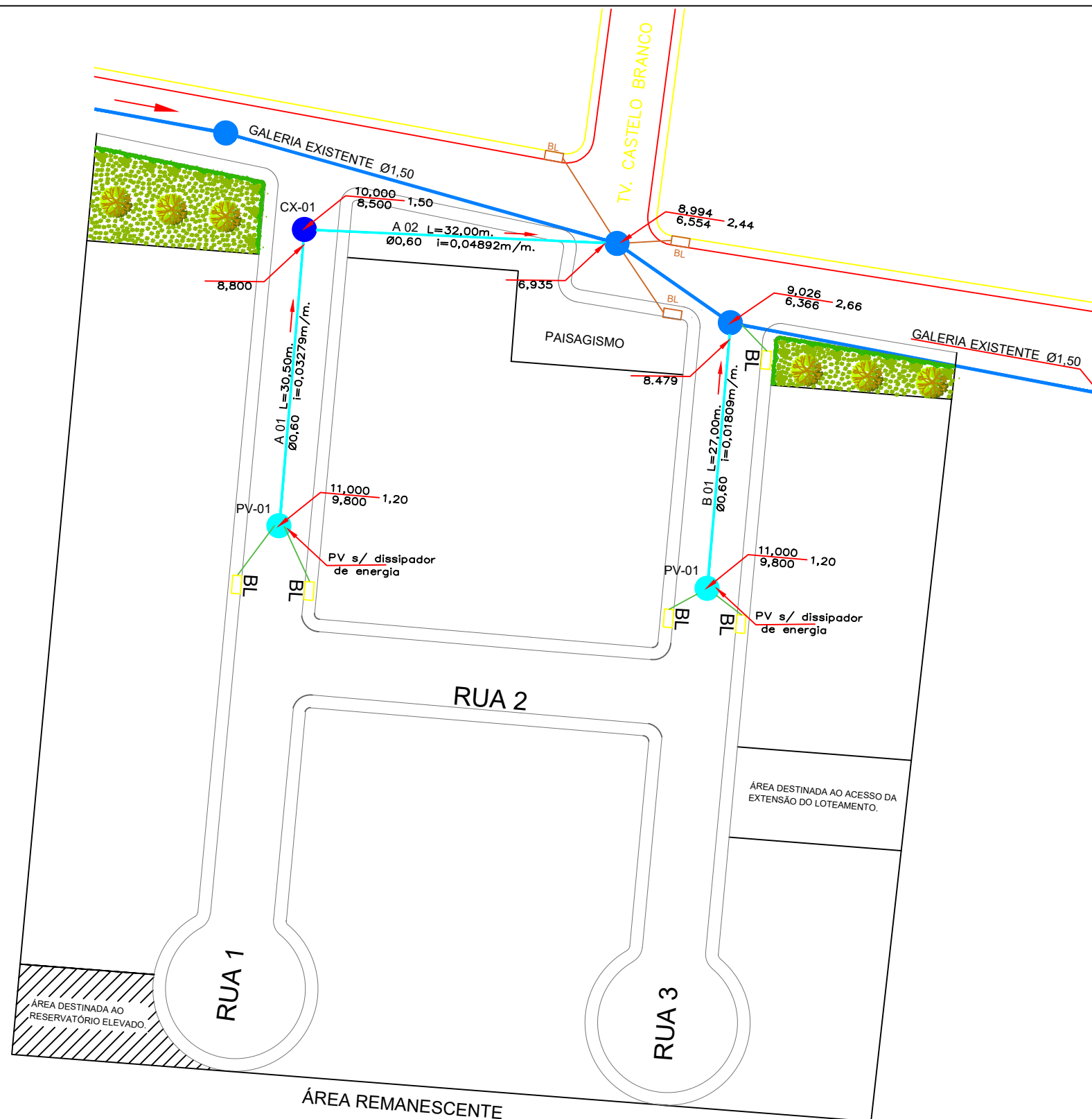
01 PLANTA GERAL - DRENAGEM
