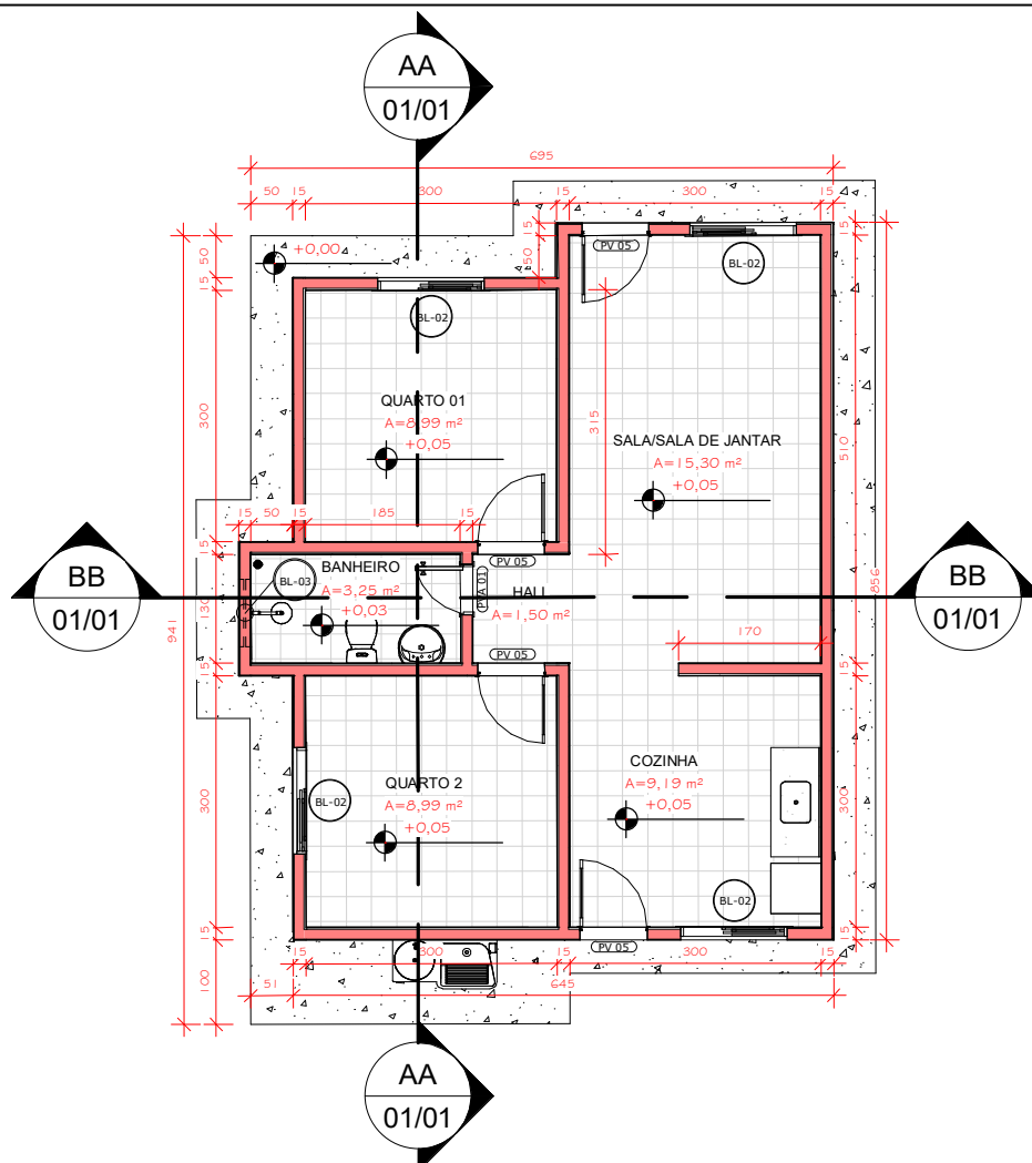
1 PAV. TÉRREO 1 : 100
