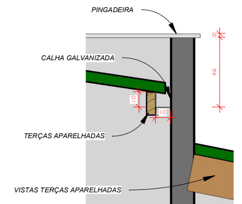
7 DET. CALHA 1 : 25
