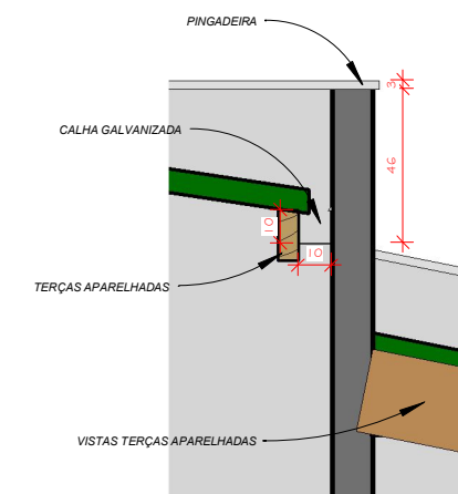
7 DET. CALHA 1 : 25
