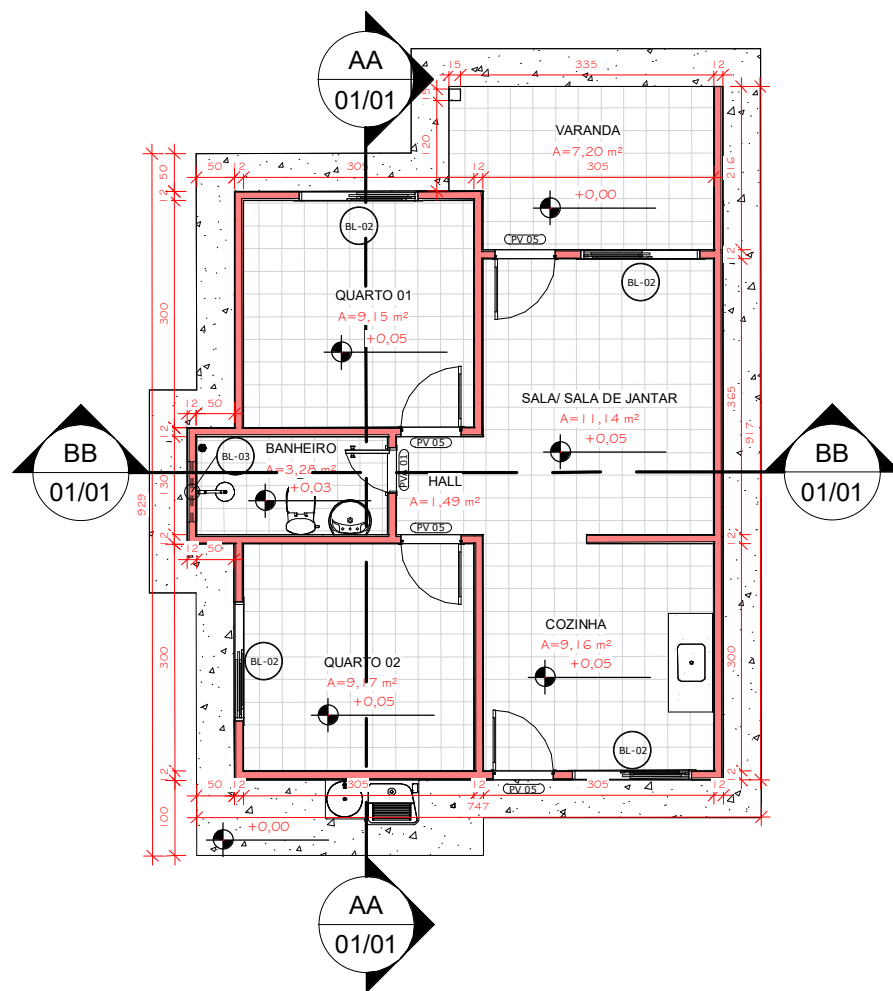
1 PAV. TÉRREO 1 : 100
