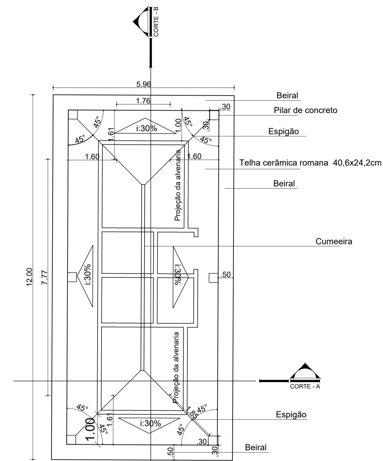
PLANTA DE COBERTURA Esc.: 1/75
