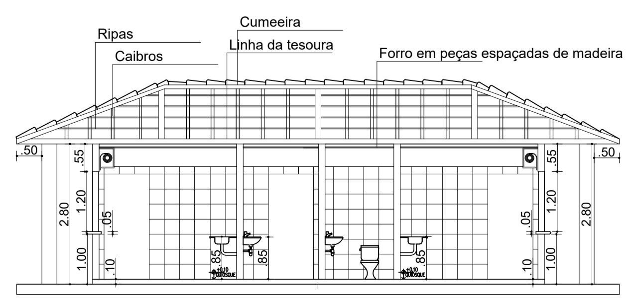
CORTE B Esc.: 1/75
