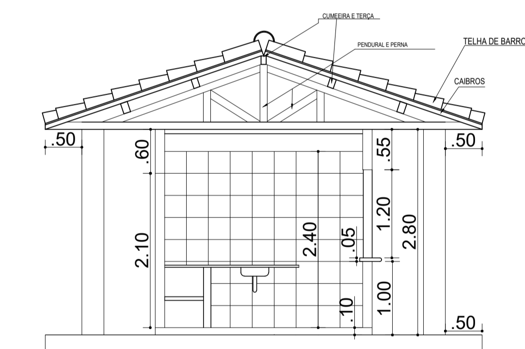
CORTE A Esc.: 1:50
