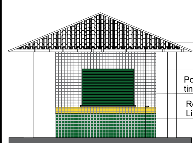
VISTA 02- LATERAL Esc.: 1/75
