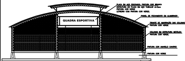
VISTA PRINCIPAL ESC.: 1/100
