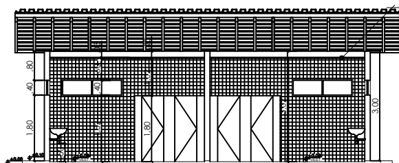
CORTE 02 (VESTIÁRIO) ESC: 1/100
