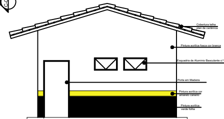
ELEVAÇÃO 01 (VESTIÁRIO) ESC: 1/100
