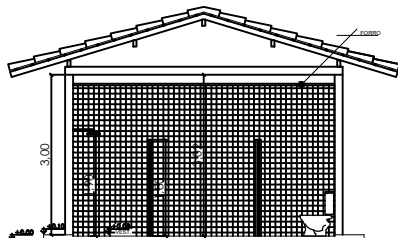
CORTE 01 (VESTIÁRIO) ESC: 1/100
