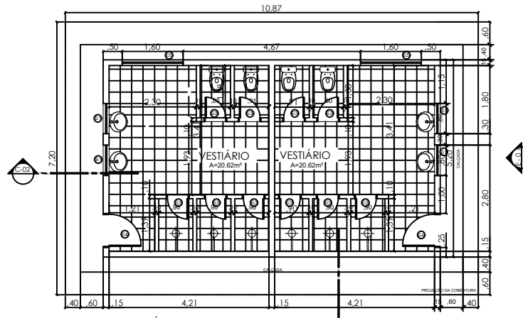
PLANTA BAIXA VESTIÁRIO ESC: 1/100
