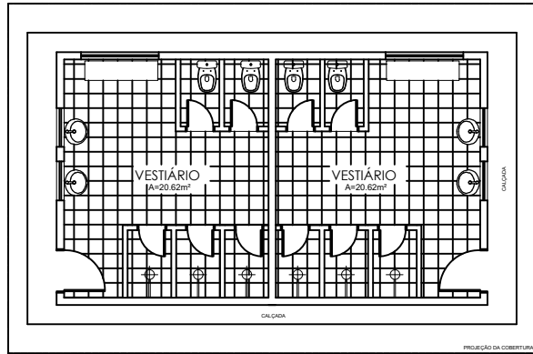
LAYOUT VESTIÁRIO ESC: 1/100
