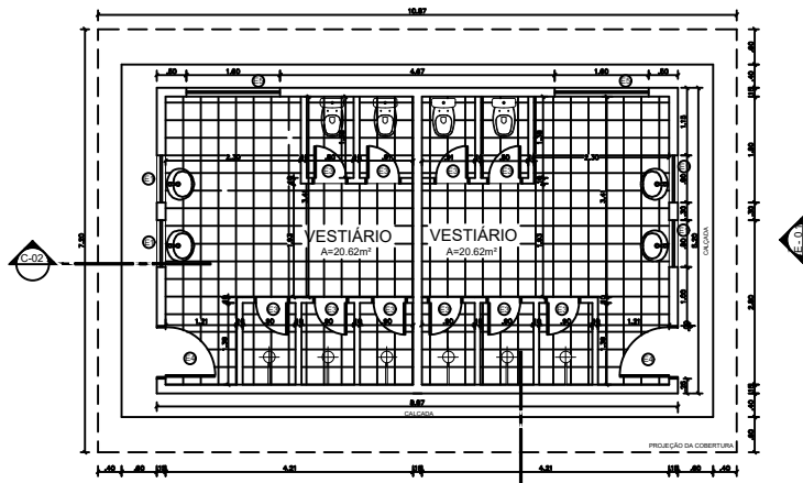
PLANTA BAIXA VESTIÁRIO ESC: 1/50
