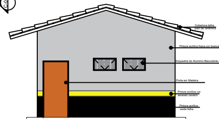
ELEVAÇÃO 01 (VESTIÁRIO) ESC: 1/50
