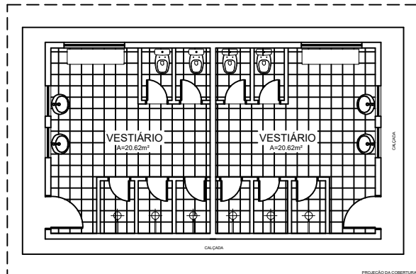
LAYOUT VESTIÁRIO ESC: 1/50
