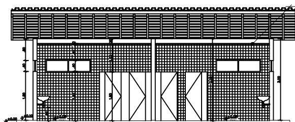
CORTE 02 (VESTIÁRIO) ESC: 1/50
