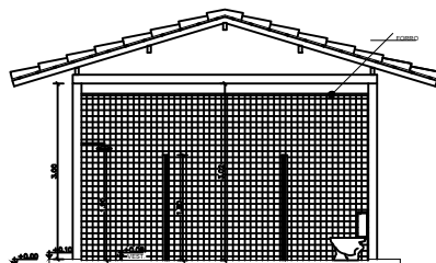
CORTE 01 (VESTIÁRIO) ESC: 1/50
