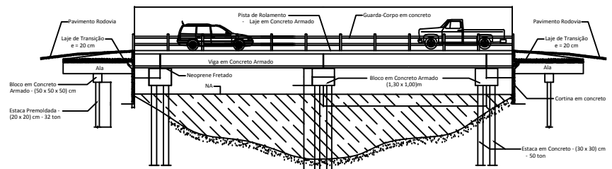
SEÇÃO 01 - LONGITUDINAL - SEM ESCALA
