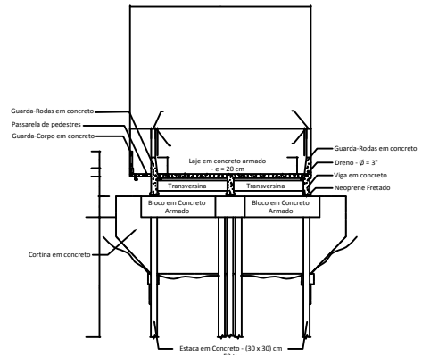
SEÇÃO 02 - TRANSVERSAL - SEM ESCALA
